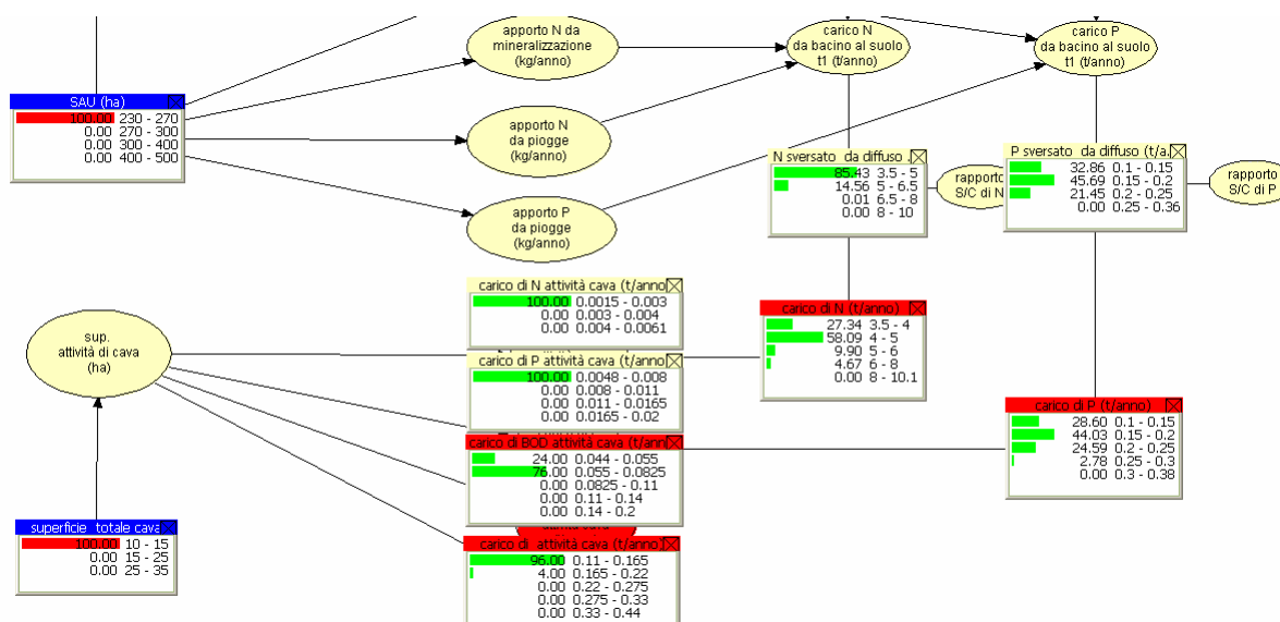
Fig 3.6-1: Modello bayesiano per la stima dei carichi inquinanti in falda
