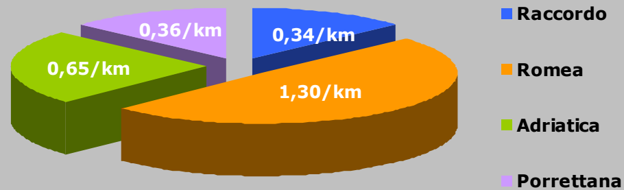
INCIDENTI MORTALI per Km nelle STRADE STATALI (2002-2012)
